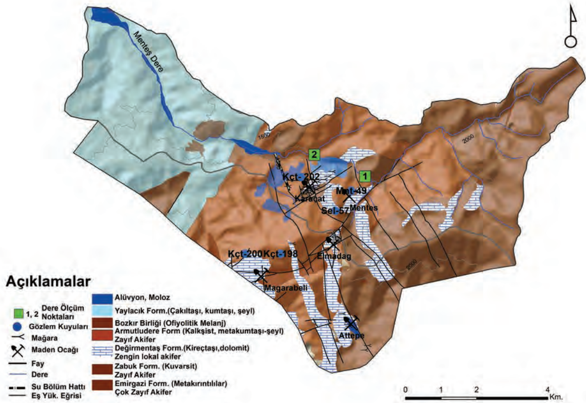
Şekil 4. İnceleme alanı hidrojeoloji haritası ve civarında açılan gözlem kuyuları (Kçt-200, Kçt-202, vb.).
